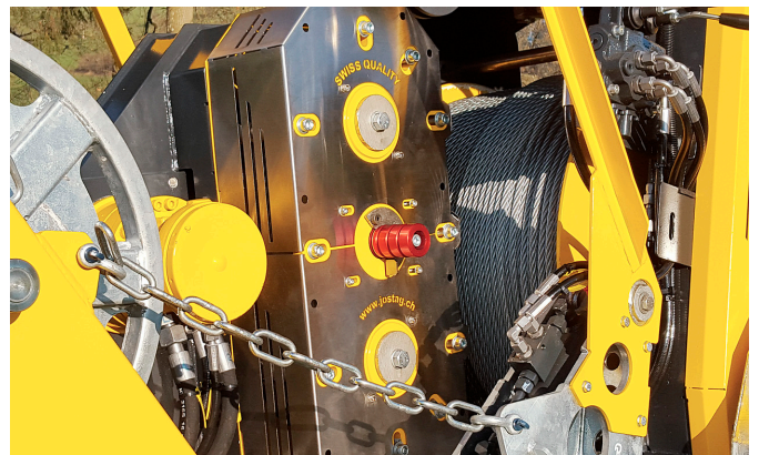
Treuil à double cabestan avec déverrouillage
